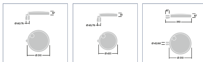
CARAT L TESTAPALO Ø 60 E Ø 76 CARAT S TESTAPALO Ø 60 E Ø 76 CARAT L LATERALE Ø 42 E Ø 60
